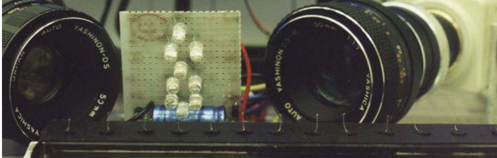
Abbildung 1.11: Bank mit Arabidopsis -Keimlingen, die nacheinander von den beiden Videokameras (nächstes Bild) dreidimensional aufgenommen werden. Infrarot-Leuchtdioden zwischen den Objektiven der Kameras zum Beleuchten der Keimlinge. /CN-bank
