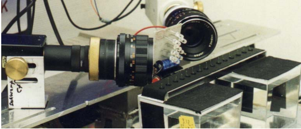
Abbildung 1.8: Eine Anlage, mit der man dreidimensionale Bilder von Arabidopsis Keimlingen aufnehmen kann. Zwei Kameras sind im rechten Winkel zueinander auf einem Schlitten montiert, der waagrecht, senkrecht und nach vorn und hinten über eine Steuereinheit bewegt werden kann. Der Ort, an dem die einzelnen Pflänzchen stehen, wird eingestellt und von der Steuerungseinheit gemerkt. Sie fährt die einzelnen Pflanzen an, macht so viel wie möglich Bilder, die gemittelt und gespeichert werden, fährt dann zu nächsten Pflanze, macht dort das gleiche, und beginnt nach vier Minuten wieder bei der ersten Pflanze. /CN-recording
