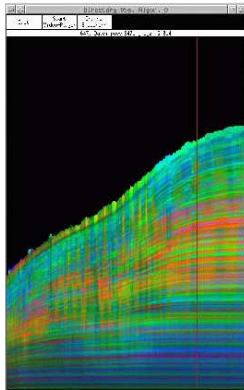
Abbildung 1.24: Farbbild vom Verlauf des Wachstums von Arabidopsis : Die nach Abbildung 1.22 erzeugten Farblinien geben die Krümmungsrichtung und -stärke am Hypokotyl in vier Minuten-Abständen wieder. Die Höhe der Linien entspricht der Länge des Hypokotyls. Die Stufen zeigen, wie stark sich der Keimling streckt: Steile Stellen entsprechen starkem Strecken, flachere geringem Strecken. Die nach rechts verlaufenden flachen oder stufenförmigen Bänder kommen durch natürliche Markierungen am oder im Hypokotyl zustande, zum Beispiel durch Unebenheiten auf der Oberfläche oder Zellgrenzen der Epidermiszellen. An ihnen kann man erkennen, welche Teile des Hypokotyls sich noch strecken (die mittleren und oberen) und welche sich nicht mehr strecken (die unteren) /diagram-cn
