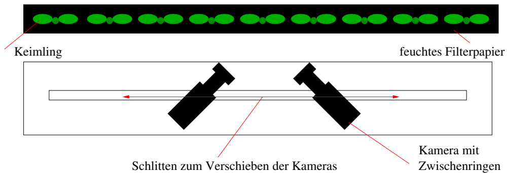
Abbildung 1.12: Zwei Videokameras werden verwendet, um dreidimensionale Aufnahmen von Arabidopsis Keimlingen zu machen. Sie werden auf einem Schlitten seitlich jeweils zur nächsten Pflanze verschoben. Am Ende fährt der Schlitten wieder an den Anfang, um nach vier Minuten wieder von jeder Pflanze Aufnahmen zu machen. /schlitten2
