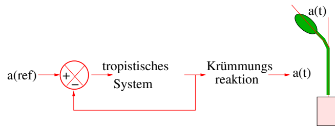
Abbildung 1.34: Rückkopplungsmodell des gravitropen Pendels. Ein Sollwert (‘senkrecht wachsen’ \alpha_{ref} ) wird mit dem Ist-Wert \alpha(t) verglichen. Wenn sich die beiden Werte unterscheiden, entsteht ein Fehlersignal e(t) . Es wird durch ein tropistisches System verstärkt und gewichtet und zeitverzögert wieder mit dem Sollwert verglichen. Rechts ist der augenblickliche Winkel \alpha(t) erklärt als Abweichung von der Lotrechten. Nach Johnsson (1977). //feedback
