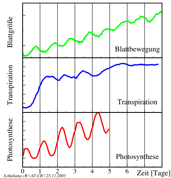
Abbildung 1.20: Circadian kontrollierte Vorgänge bei Arabidopsis : Oben: Größenzunahme des Primärblattes (grüne Kurve). Mitte: Transpiration (blaue Kurve). Unten: Photosynthese (rote Kurve). Hierbei wurde die rhythmische Regulation eines wichtigen Gens der Photosynthese (LHC = light harvesting complex oder Antennenpigment) mit einem genetischen Trick gemessen: Die Genexpression kann durch Biolumineszenz verfolgt werden. /cr-arabidopsis
